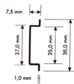
Profil 4000
