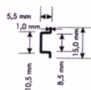
Profil 4004
