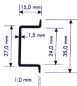
Profil 4006
